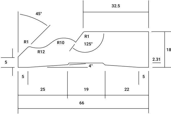
COLONIAL AS2 66mm x 18mm
