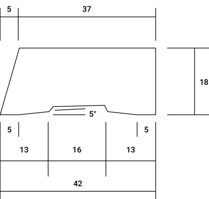
BEVEL AS3 42mm x 18mm
