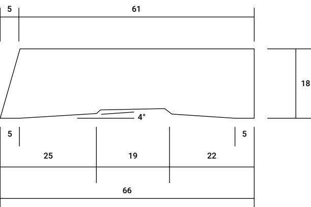
BEVEL AS3 66mm x 18mm
