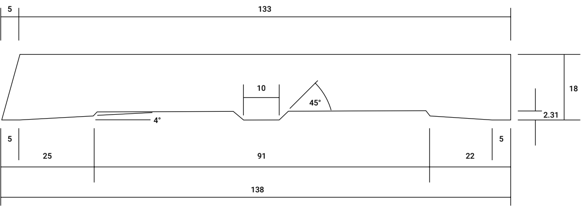
BEVEL AS3 138mm x 18mm
