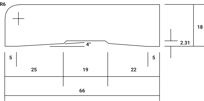
PENCIL ROUND AS7 66mm x 18mm
