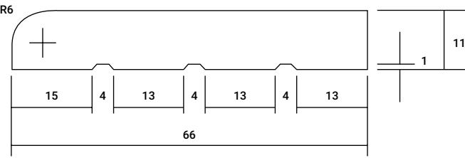
PENCIL ROUND AS15 66mm x 11mm
